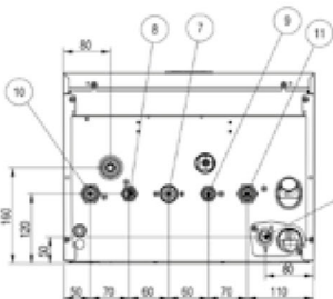
VISTA INFERIORE
