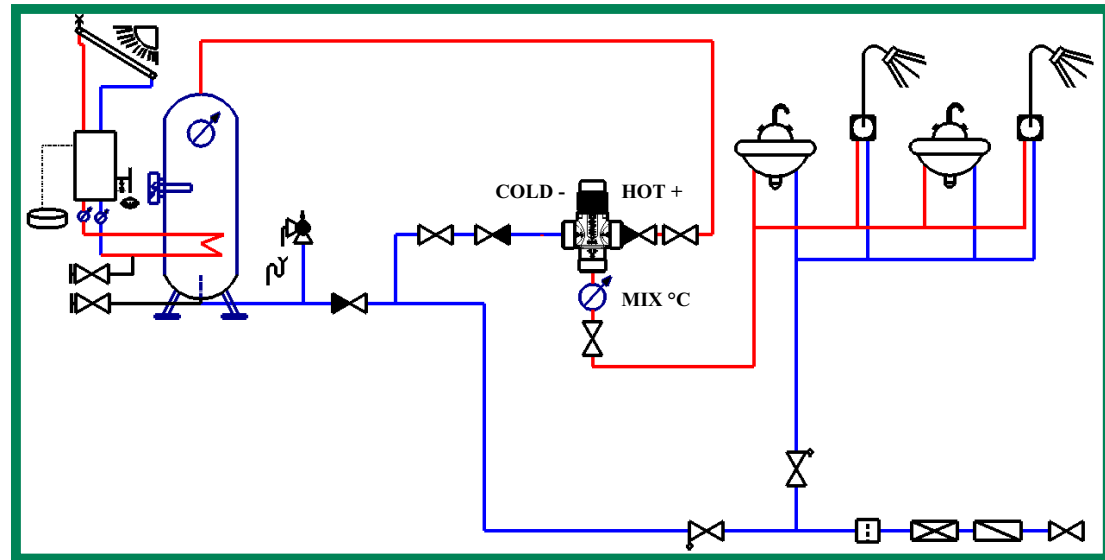
Fig 3: Esempio applicativo di RA / Fig. 3: RA application example / Abb. 3: Anwendbares Beispiel von RA / Dessin 3: exemple d'application de RA / Fig 3: Ejempolos aplicativo de RA
