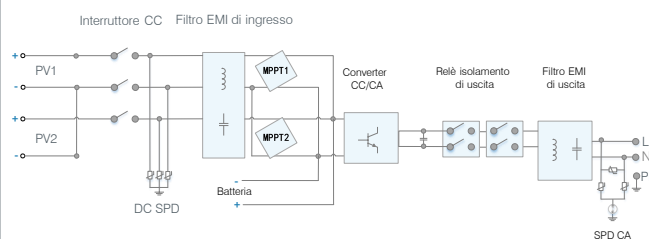
Schema elettrico
